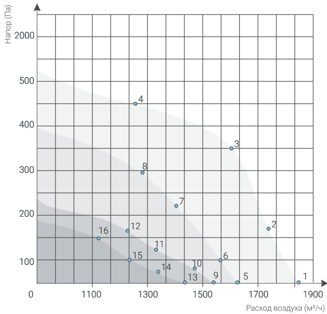
Данные измерений
