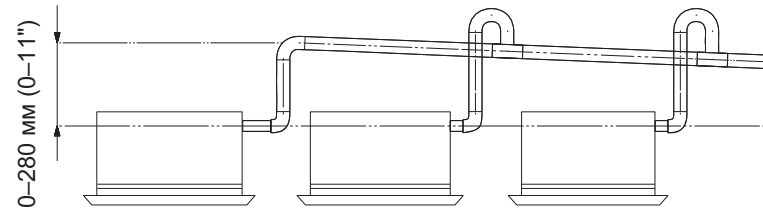
Т-образное соединение дренажных труб
