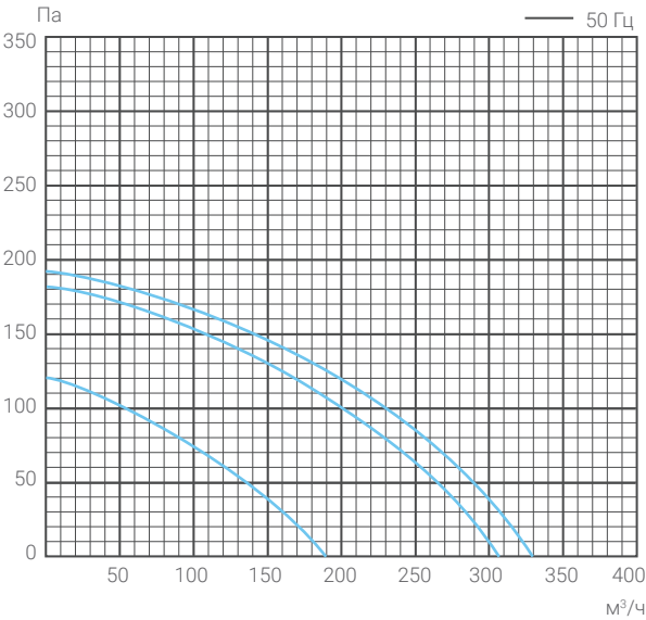
LV-PACU-600-P-AC-WiFi-E50
