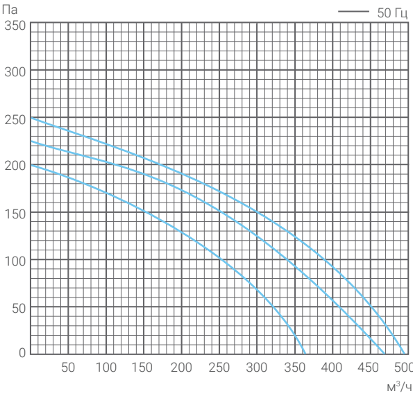
LV-PACU-800-P-AC-WiFi-E50
