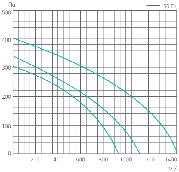
LV-PACU-1200-P-AC-WiFi-E50
