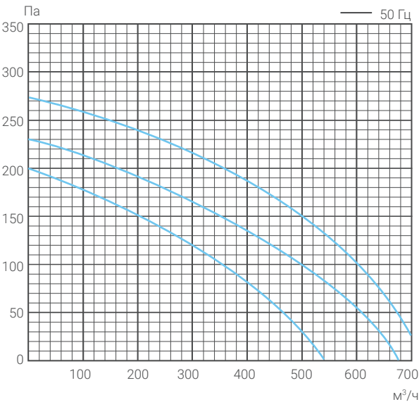
LV-PACU-1000-P-AC-WiFi-E50
